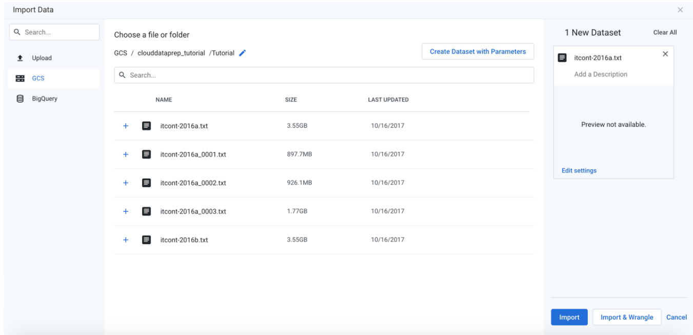
Figure: Browser
